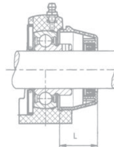
Couvercle plastique pour palier à semelle + joint
