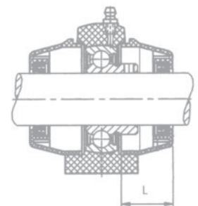
Couvercle plastique pour palier à semelle + joint
