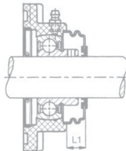
Couvercle inox pour palier applique + joint arrière
