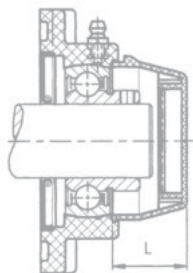
Couvercle plastique pour palier applique + joint arrière
