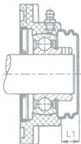
Couvercle inox pour palier applique + joint arrière
