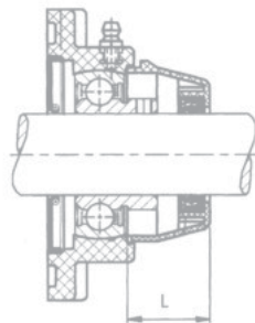
Couvercle plastique pour palier applique + joint arrière
